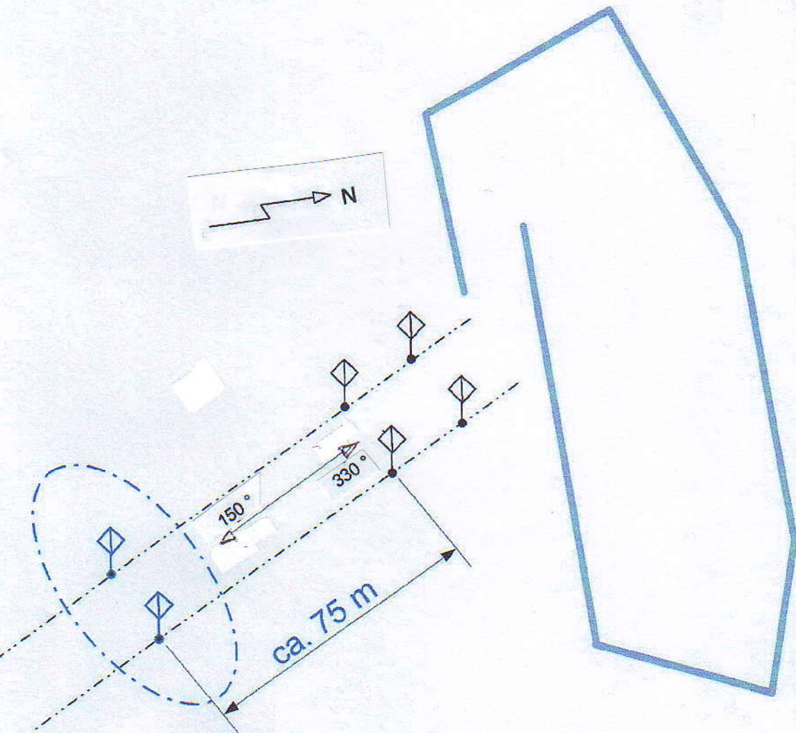
2 zusätzliche Dalben in Verlängerung der bisherigen Einfahrtsdalben
